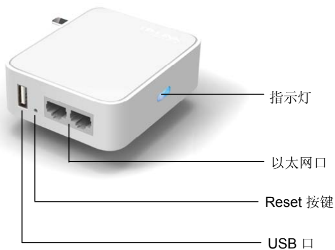
图 3-1 TL-WR720N 外观图
